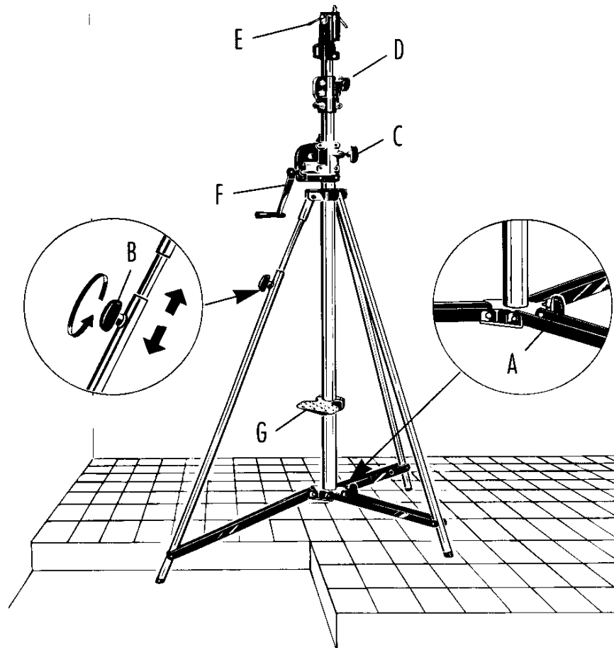
Abbildung 1: Aufstellhinweise
