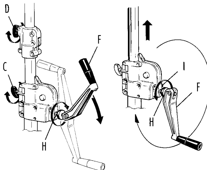
Abbildung 3: Höhenverstellung des Stativs
